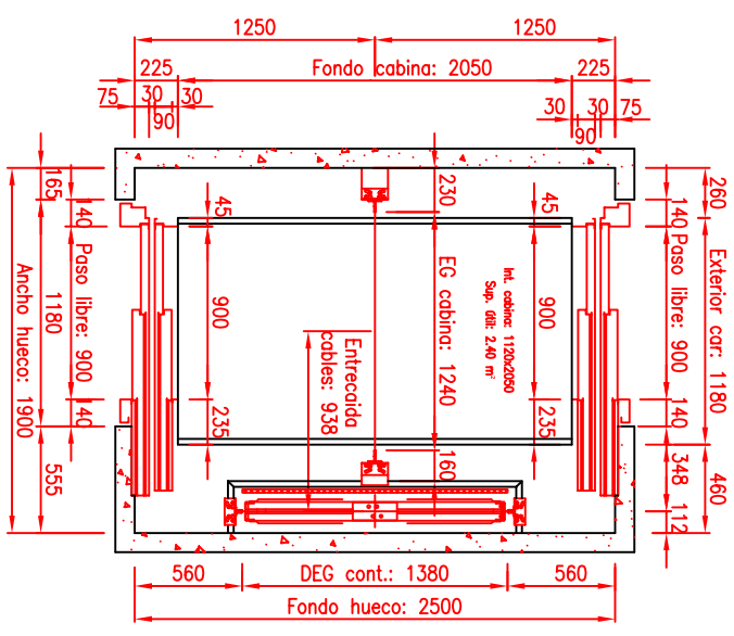
PLANTA HUECO
