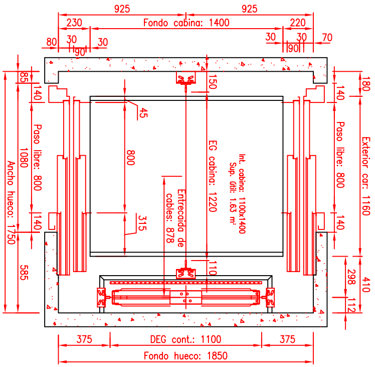
PLANTA HUECO
