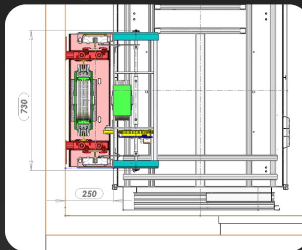
Detalle planta
