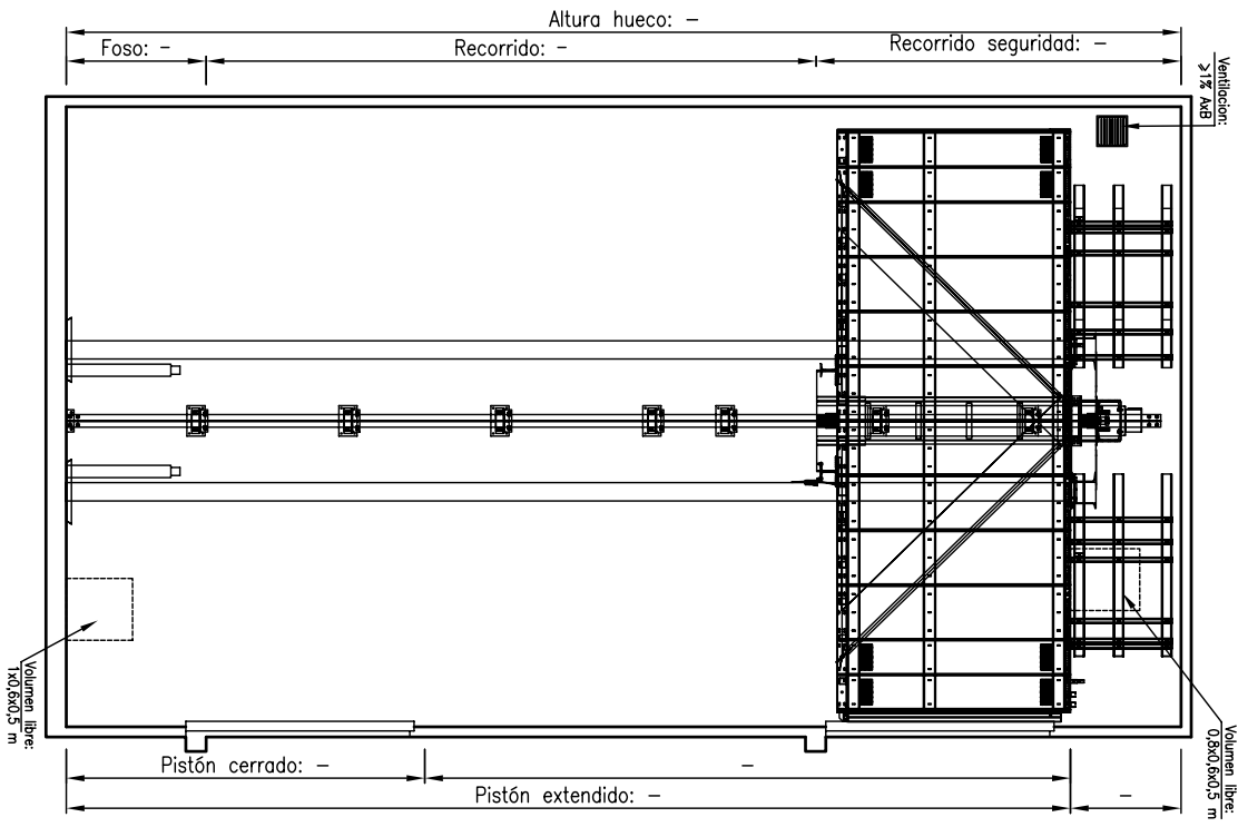
SECCION VERTICAL
