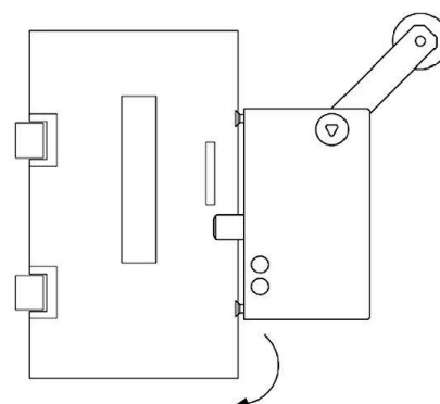
CERRADURAS DERECHAS (VISTO DESDE EL RELLENO) RIGHT SAFETY LOCK (SEEN FROM FLOOR) SERRURES DROITES (VUES DE L'ÉTAGE)
