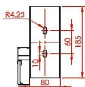
Soporte / Bracket
