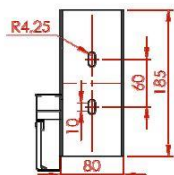
Soporte / Bracket
